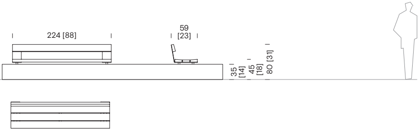
Banc d'un tronçon avec dossier sur muret BSB+114
