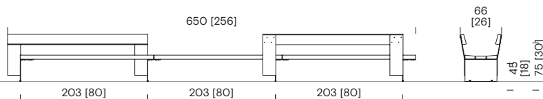
Banc de trois tronçons avec trois dossiers BCB+314
