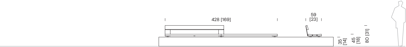
Banc d'un tronçon sans dossier sur muret BSB+104
