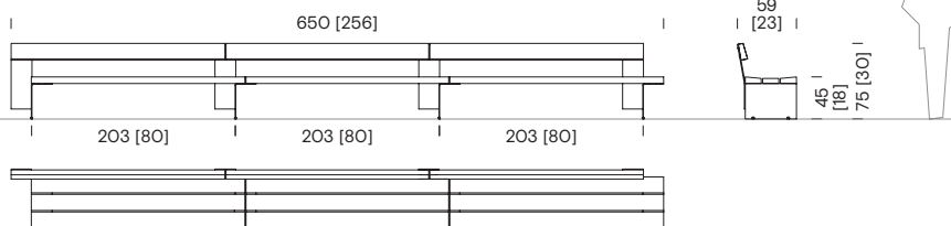
Banc de trois tronçons avec trois dossiers BCB+314
