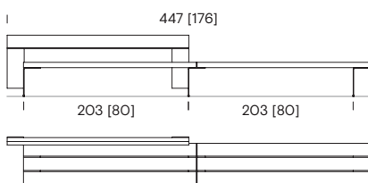
Banc de deux tronçons avec un dossier BCB+204
