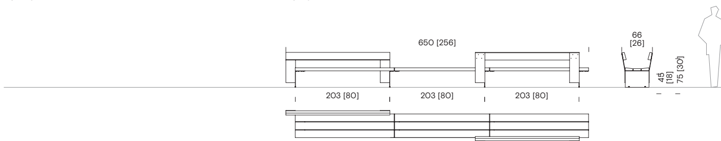
Banc de trois tronçons deux dossiers inversés avec BCB+304
