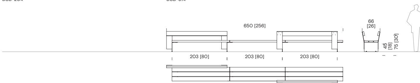
Bank mit drei Abschnitten und zwei umgekehrten Rückenlehnen BCB+304
