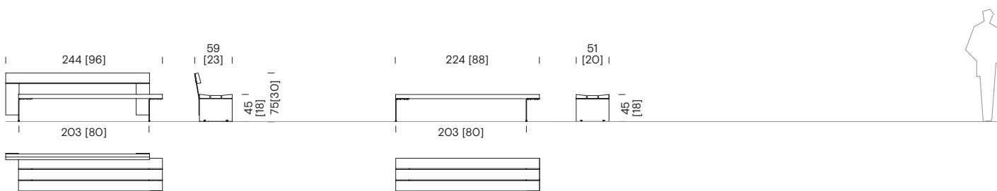
Bank mit einem Abschnitt und Rückenlehne BCB+114
