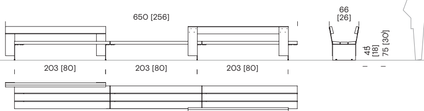
Bank mit drei Abschnitten und zwei umgekehrten Rückenlehnen BCB+304
