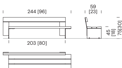
Bank mit einem Abschnitt und Rückenlehne BCB+114
