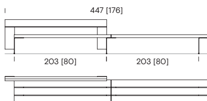
Bank mit zwei Abschnitten und einer Rückenlehne BCB+204
