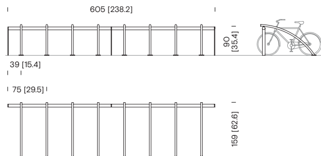
Fahrradständer mit zwei Abschnitten BIA+211
