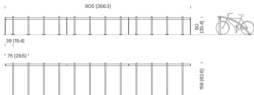
Fahrradständer mit drei Abschnitten BIA+311
