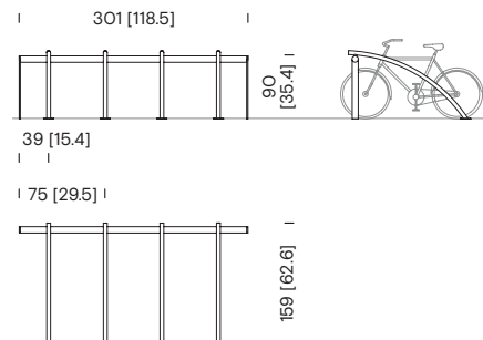
Fahrradständer mit einem Abschnitt BIA+111
