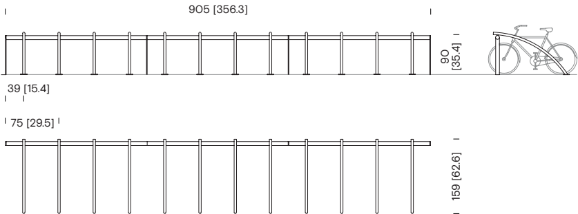
Parc à vélos de trois tronçons BIA+311
