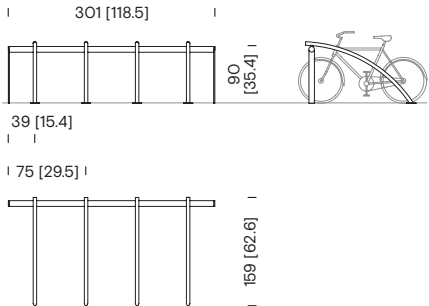
Parc à vélos d'un tronçon BIA+111
