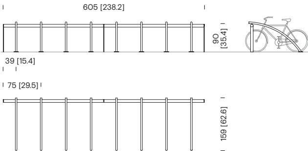
Parc à vélos de deux tronçons BIA+211
