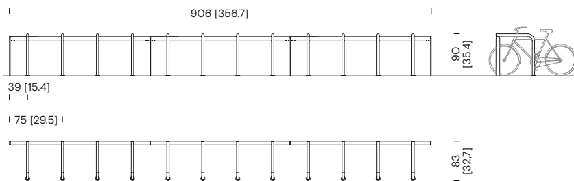
Fahrradständer mit drei Abschnitten BIA+321
