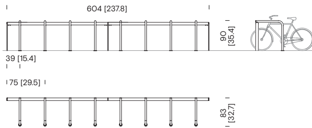
Fahrradständer mit zwei Abschnitten BIA+221
