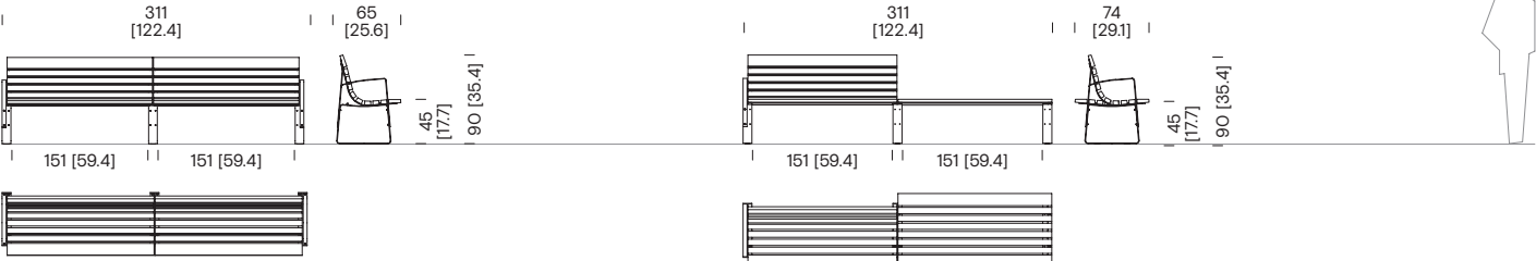
Banc de deux tronçons avec deux dossiers et deux bras BLB+214
