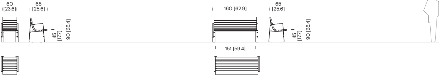
Banc d'un tronçon avec dossier et deux bras de 0,60 m BLB+004
