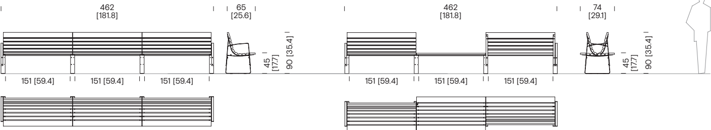
Banc de trois tronçons avec trois dossiers et deux bras BLB+314
