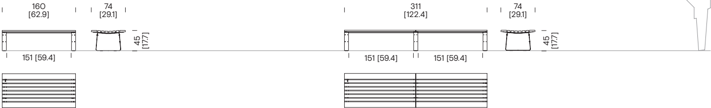
Banc d'un tronçon sans dossier BLB+104
