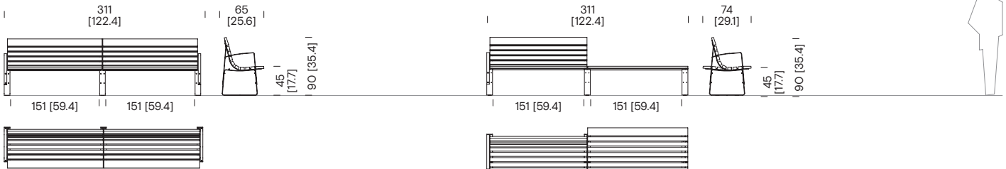
Bank mit zwei Abschnitten, zwei Rückenlehnen und zwei Armlehnen BLB+214
