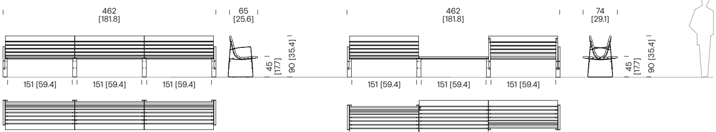
Bank mit drei Abschnitten, drei Rückenlehnen und zwei Armlehnen BLB+314
