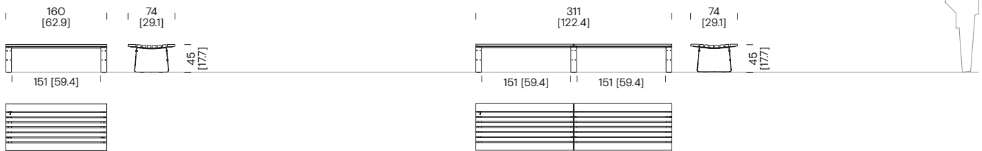
Bank mit einem Abschnitt ohne Rückenlehne BLB+104
