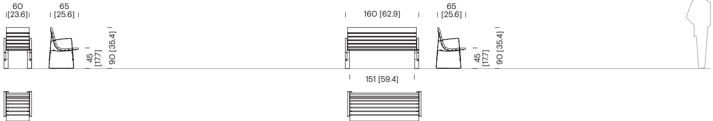
Bank mit einem Abschnitt, Rückenlehne und zwei Armlehnen; 0,60 m BLB+004
