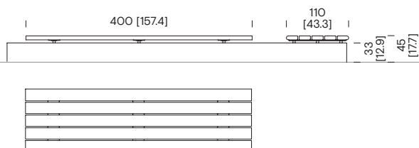
Banc de 4 m sans dossier sur muret CSB51
