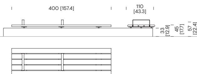
Banc de 4 m sans dossier sur muret CSB51
