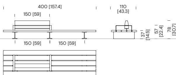
Banc de 4 m avec dossier COB52
