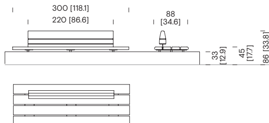
Banc de 3 m avec dossier sur muret CSB42
