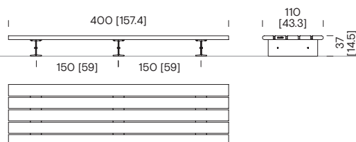
Banc de 4 m sans dossier COB51
