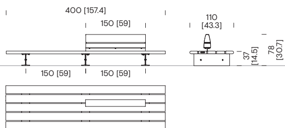
Banc de 4 m avec dossier COB52
