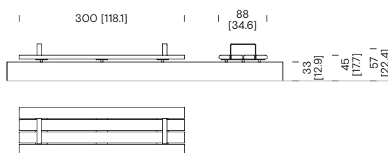
Banc de 3 m sans dossier sur muret CSB41
