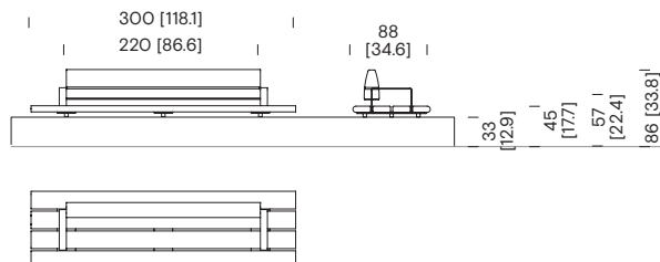
Banc de 3 m avec dossier sur muret CSB42
