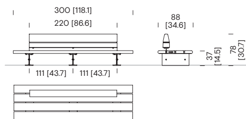
Banc de 3 m avec dossier COB42
