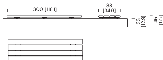
Banc de 3 m sans dossier sur muret CSB41
