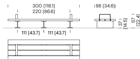
Banc de 3 m sans dossier COB41
