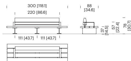
Banc de 3 m avec dossier COB42
