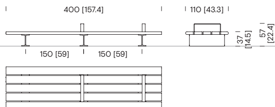
Banc de 4 m sans dossier COB51
