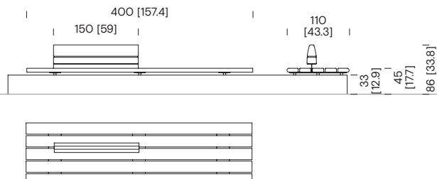
Banc de 4 m avec dossier sur muret CSB52
