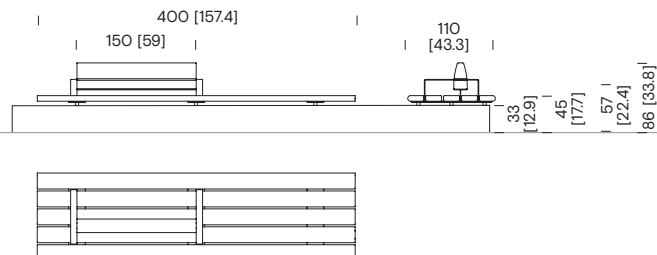
Banc de 4 m avec dossier sur muret CSB52
