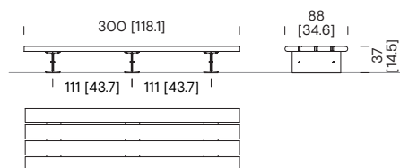
Banc de 3 m sans dossier COB41
