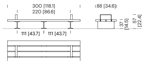
Bank 3 m ohne Rückenlehne COB41
