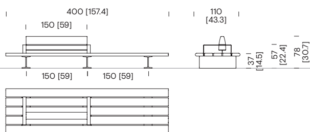
Bank 4 m mit Rückenlehne COB52
