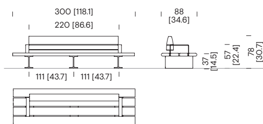
Bank 3 m mit Rückenlehne COB42
