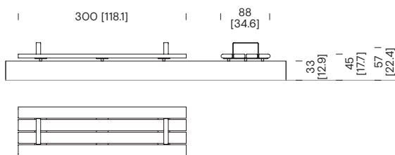
Bank 3 m ohne Rückenlehne an Mauer CSB41
