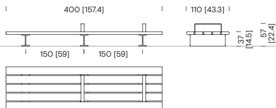
Bank 4 m ohne Rückenlehne COB51
