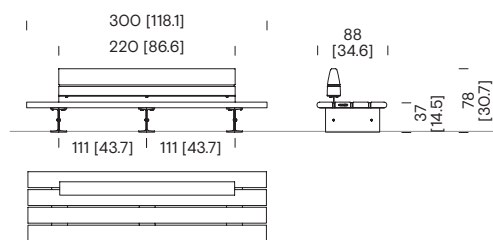
Bank 3 m mit Rückenlehne COB42
