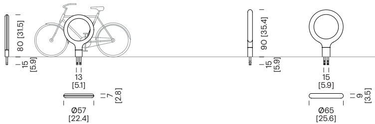
Fahrradständer Ø 57
