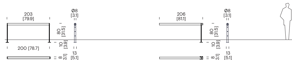
Geländer mit einem Abschnitt
