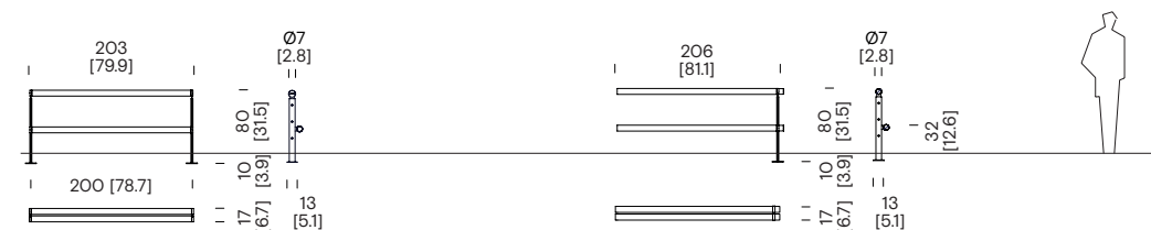
Bank mit einem Abschnitt und Querstange
