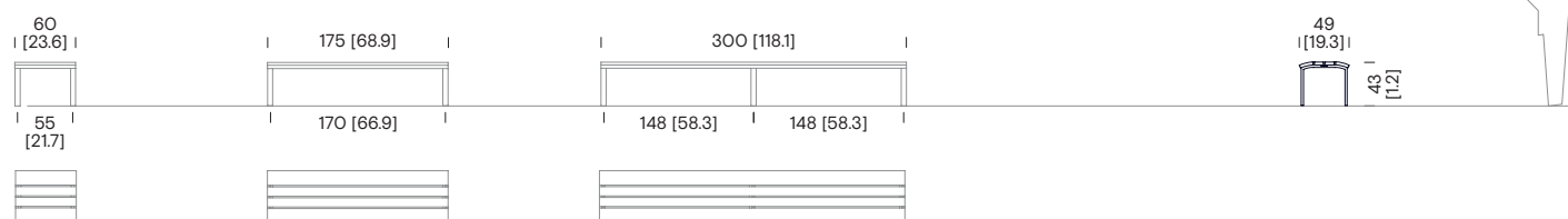
Hocker 0,60 m
