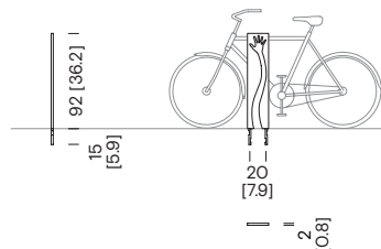
Fahrradständer TAP11
