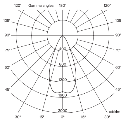
Simétrica Distribución Flood LOR 100% ULOR 0%±3%
