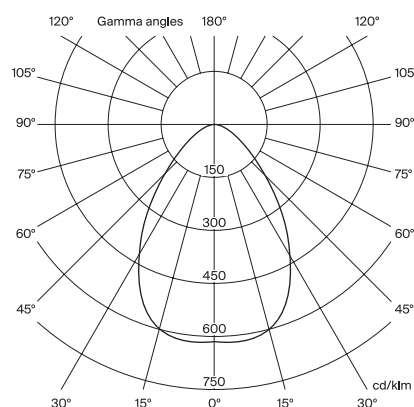
Simétrica Distribución W. Flood Opal LOR 100% ULOR 0%±3%
